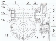
Obr. 17.2 Náhradní díly MRP
