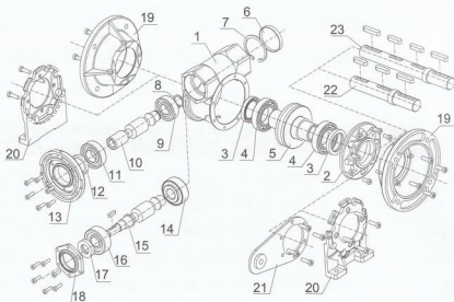
Obr. 17.1 Náhradní díly MRT
