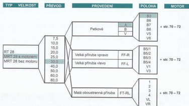
Schéma typového značení
